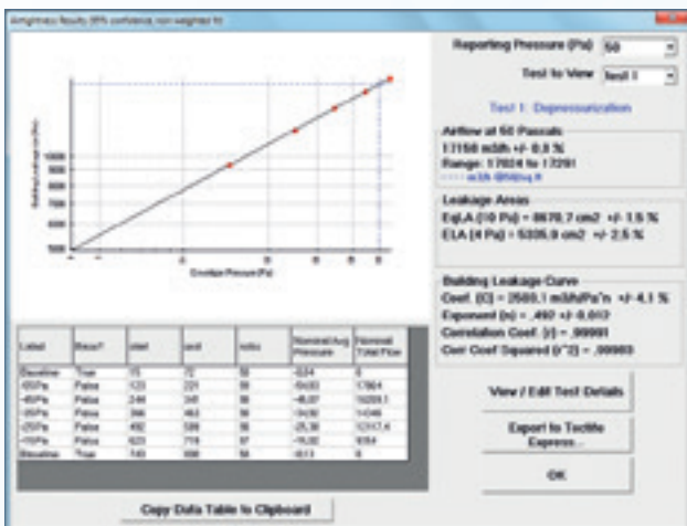
Leckagekurve mit Volumenstrom-Ergebnissen
