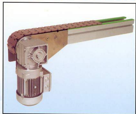
Antriebstation mit Aufsteckgetriebe (Hohlwelle), 300 mm lang, Bauhöhe 160 mm
