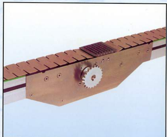
Stirnseitige Übergabestation, 570 mm lang, Bauhöhe 160 mm
