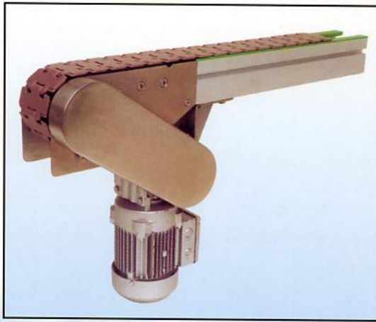
Antriebstation mit Kettentrieb, 300 mm lang, Bauhöhe 160 mm
