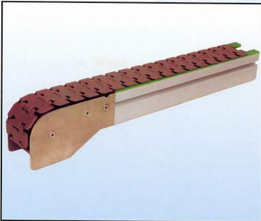
Umlenkstation, 220 mm lang, Bauhöhe 130 mm
