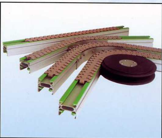
Aluminium-Bandkörper, Bauhöhe 80 mm
