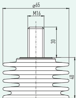
F6 M16x30
