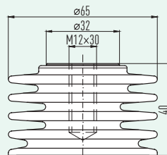
F6 iM12x30
