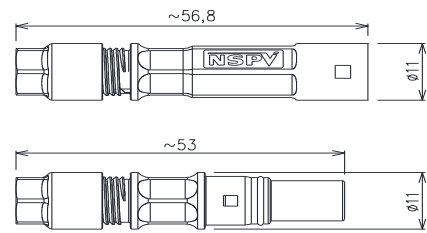
Newsun 1000VDC Mini cable connector:
